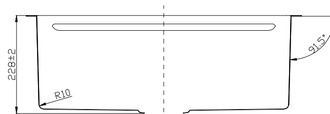
剖面 A-A
