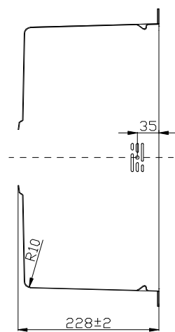
剖面 B-B
