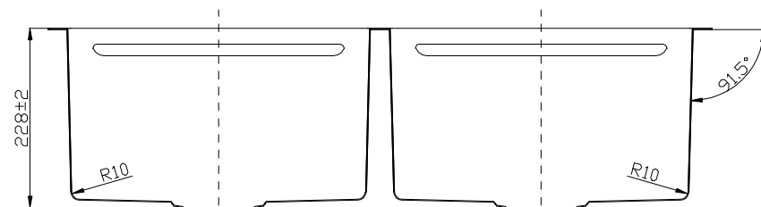
剖面 A-A
