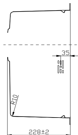
剖面 B-B
