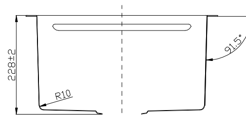
剖面 A-A
