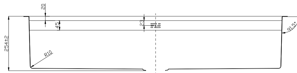
剖面 A-A
