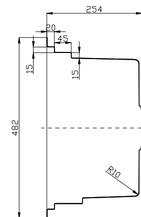
剖面 B-B
