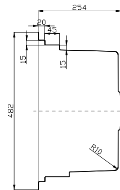
剖面 B-B
