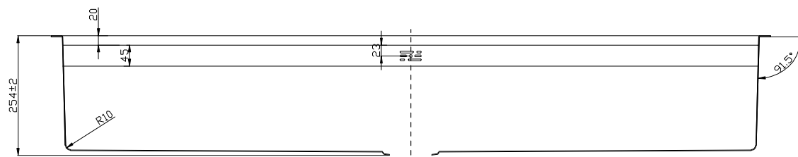
剖面 A-A
