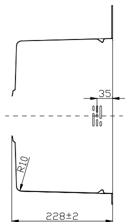
剖面 B-B
