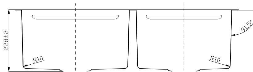
剖面 A-A
